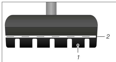
Obr.: Brzdová čelist s indikátorem opotřebení (ilustrační příklad)
